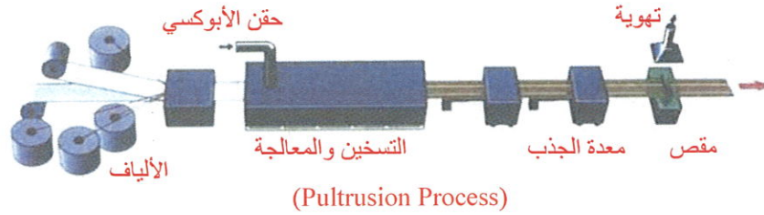
شكل رقم ٢. إحدى طرق تصنيع المواد البوليمرية المسلحة بالألياف
