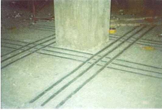
تدعيم السقف في منطقة عزوم الإنحناء السالبة
