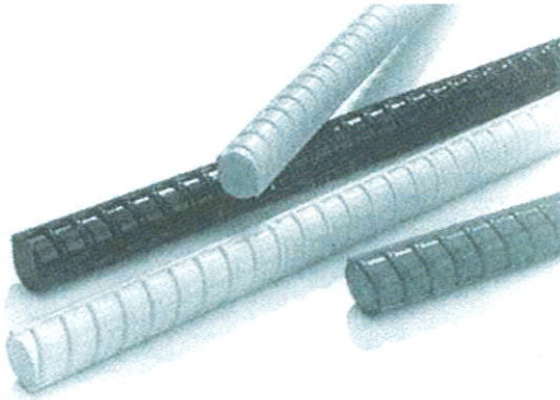
قضبان المواد البوليمرية المسلحة بألياف الزجاج
